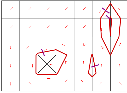
Fig. 8. Semi-separatrices.
