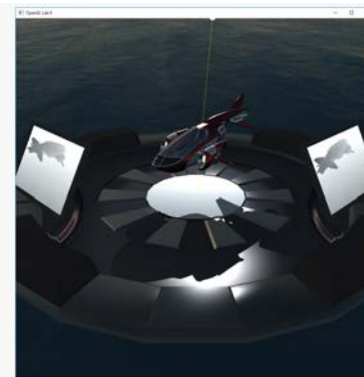
Shadow maps
