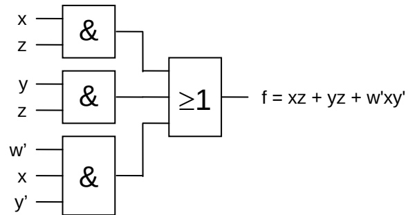
Figur 3.13 OCH/ELLER (AND/OR)-nät.
