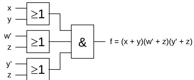
Figur 3.14 ELLER/OCH (OR/AND)-nät.
