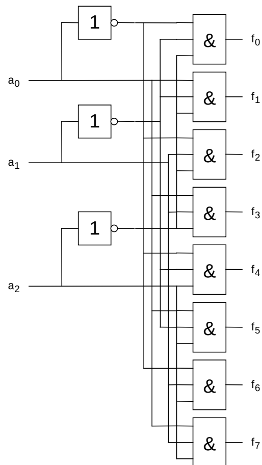
Figur 4.10 Prosamsymbol för "NBC till en av åtta" ("Binary/Octal") kodomvandlare.
