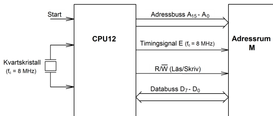
Figur 13.6 CPU12 kopplad till minnet (adressrum M).
